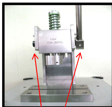
レバーは左右取り付け可能
