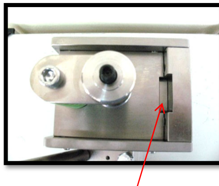
研磨によるスライドキー
