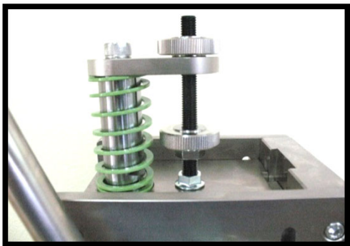
ストロークが簡単に調整可能
