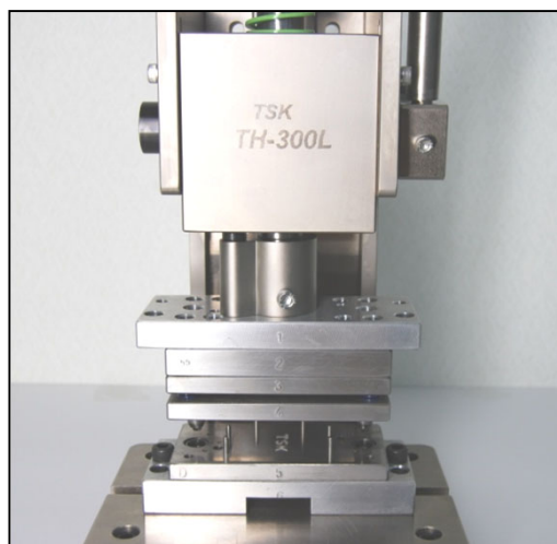
研磨によるスライドキー
